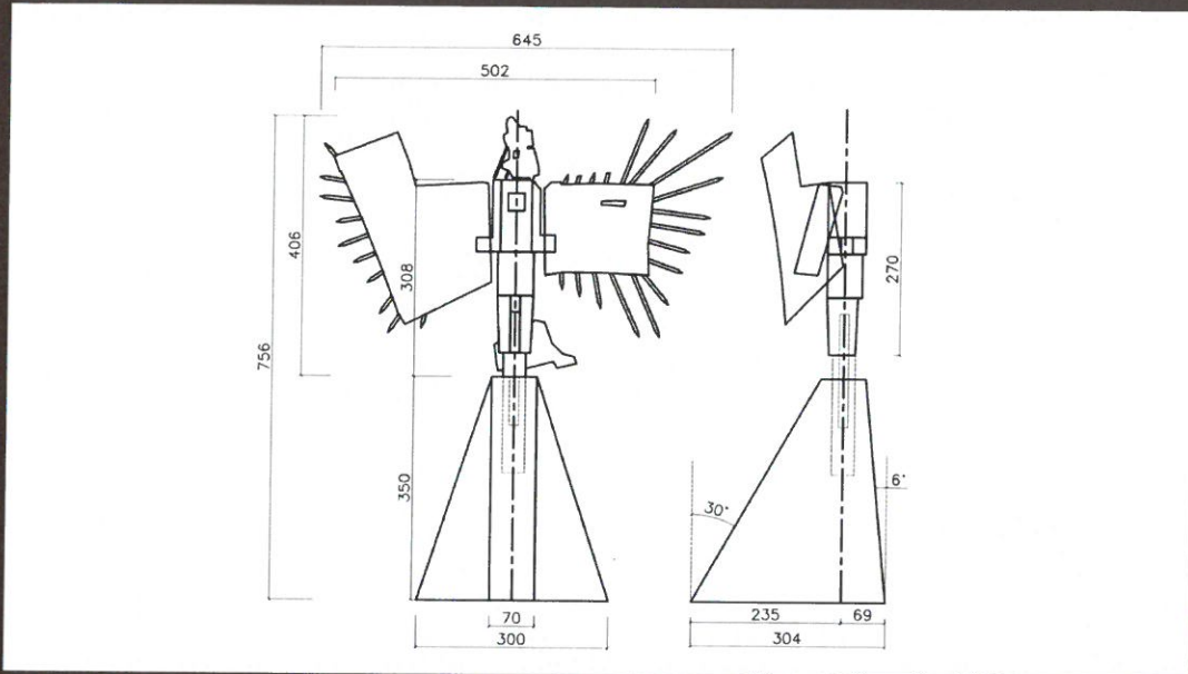
RYSUNEK POMNIKA - GABARYTY
